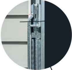
Stabiles drei Federsystem
